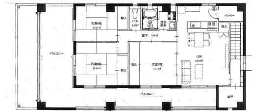
医師住宅 間取り
